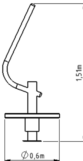
DIMENSÕES
