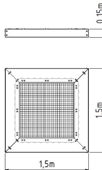
DIMENSÕES
